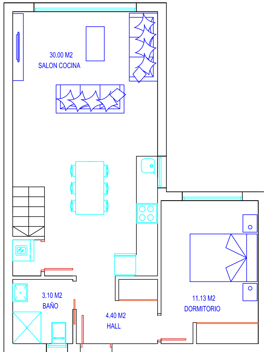
planta baja
